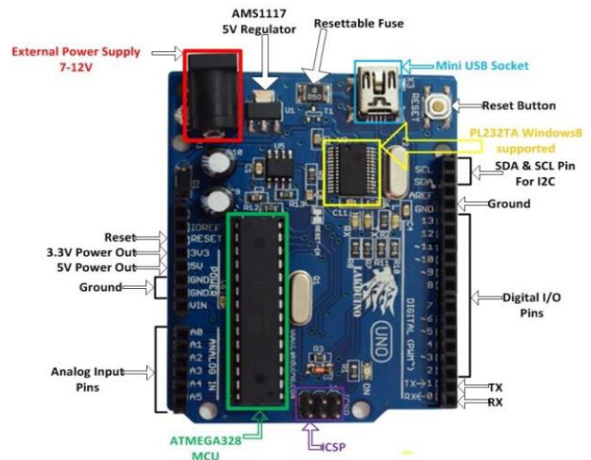
Fig.5. Arduino uno
